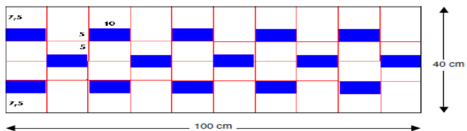
DISTRIBUCIÓN HABITUAL DE LOS MÓDULOS DE RESALTE EN BANDAS TRANSVERSALES DE ALERTA
