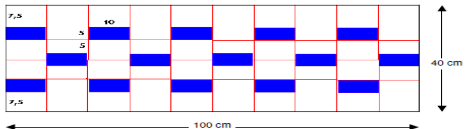
DISTRIBUCIÓN HABITUAL DE LOS MÓDULOS DE RESALTE EN BANDAS TRANSVERSALES DE ALERTA
